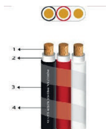
Cable N2XOH INDECO
